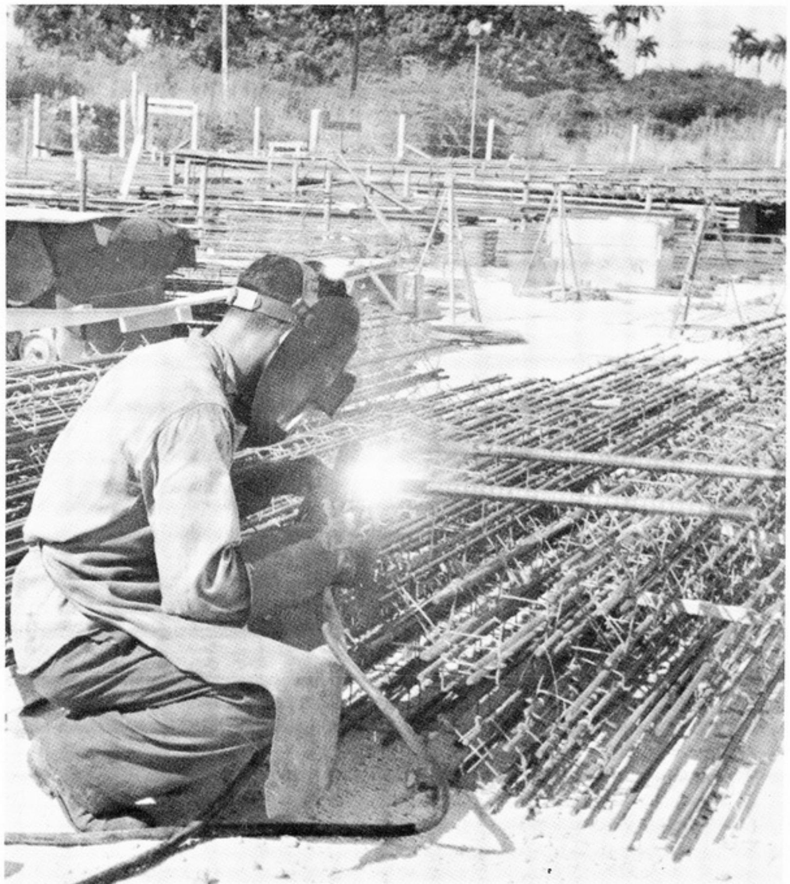
Invariablemente todo el encabillado se suelda previamente para evitar surja cualquier falla.
