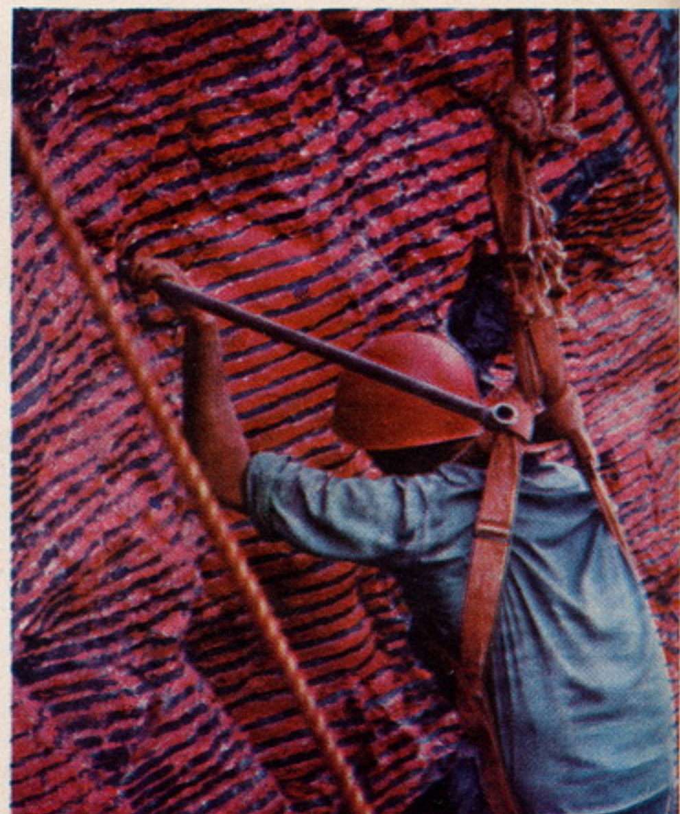
Se mantiene la roca seca canalizando las filtraciones de agua por medio de unos tubos.
